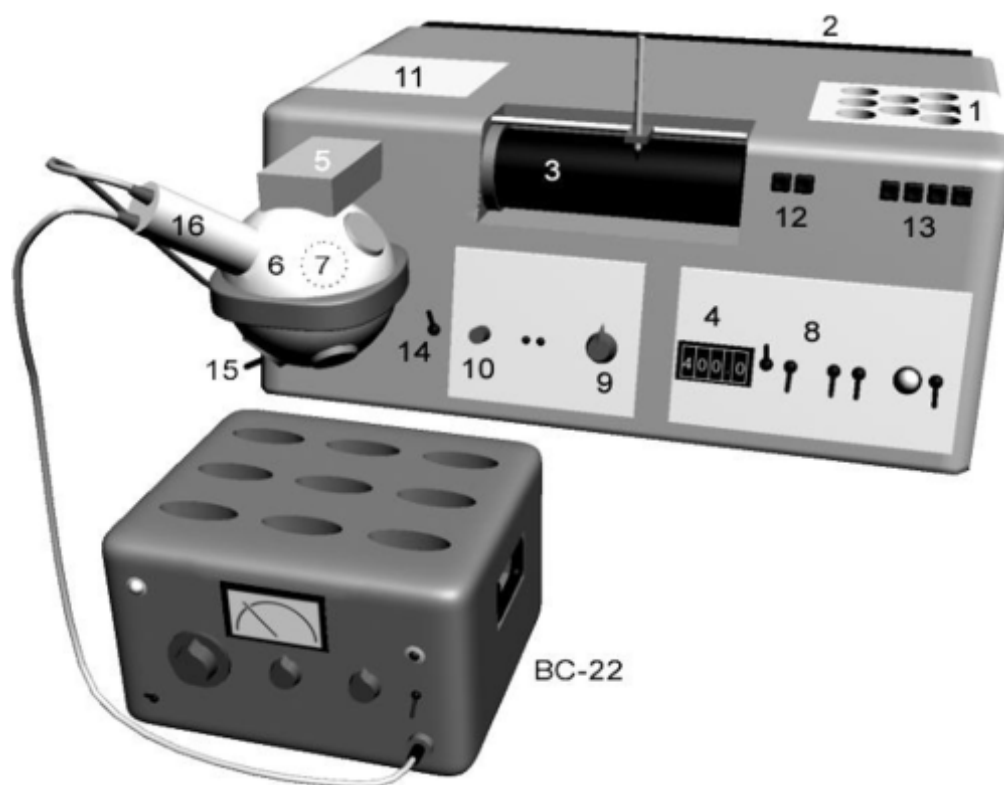
Рис. 3. Вигляд спектрофотометра СФ-181С з боку передньої панелі. 1 – кришка доступу до лампи та вхідної щілини; 2 – монохроматор; 3 – самописець; 4 – лічильник довжин хвиль (в ангстремах); 5 – кюветне відділення; 6 – інтегруюча сфера Ульбріхта; 7 – фотоелемент Ф-10; 8 – пульт управління приладом; 9 – рукоятка «Підсилення»; 10 – запобіжник; 11 – кришка доступу до перемикача Д і Т та вихідної щілини; 12 – перемикач сполучення барабана самописця і лічильника довжин хвиль; 13 – перемикач швидкостей розгортки спектра; 14 – модулятор-переривач; 15 – перемикач "Ф-10-ФЕП"; 16 – фотопомножувач ФЕП-28 у захисному кожусі.
