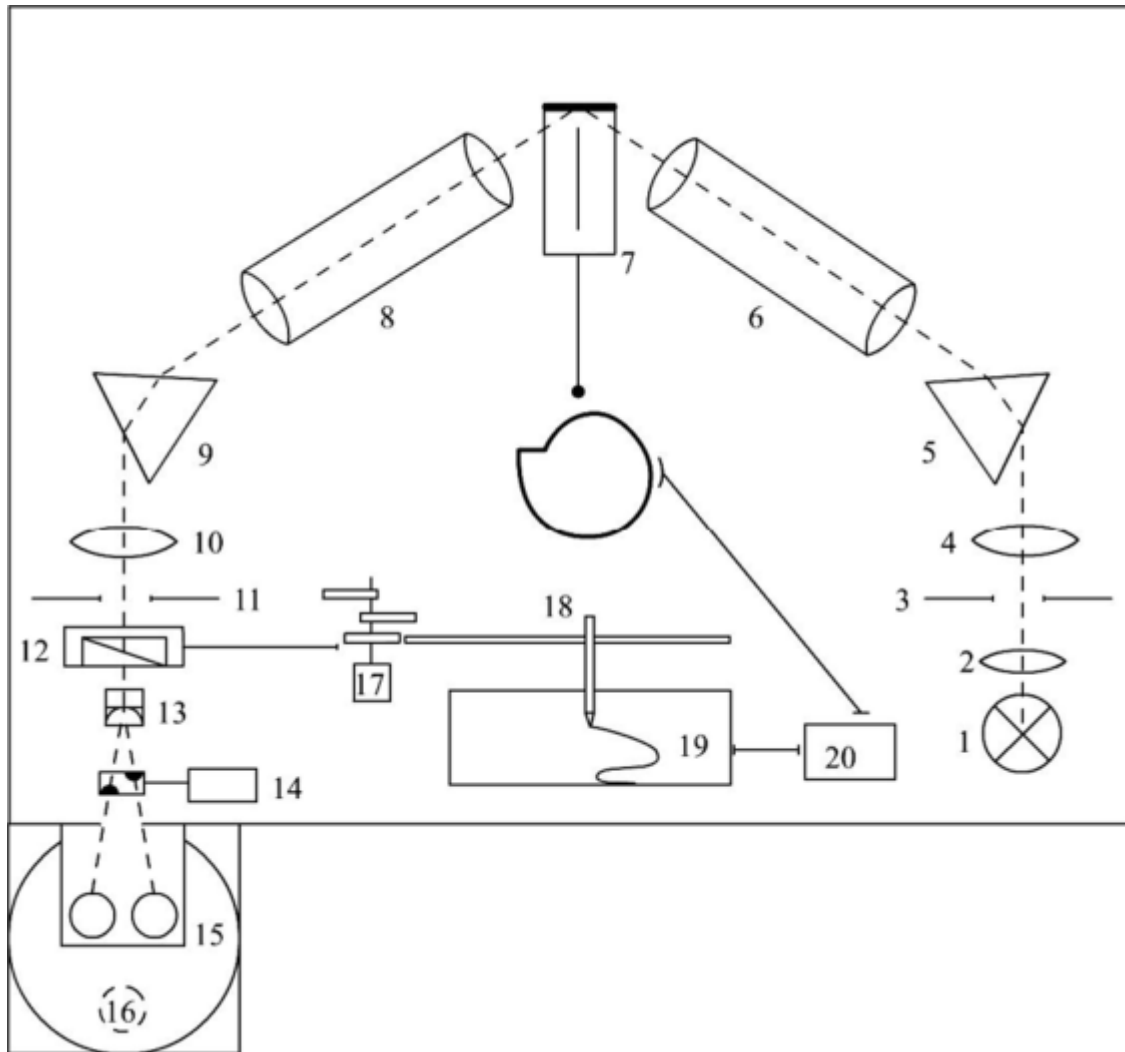
Рис. 2. Оптико-механічна схема реєструючого спектрофотометра СФ-18ІС: 1 – джерело світла (лампа розжарювання); 2 – лінза-конденсор; 3 – вхідна щілина монохроматора; 4 – лінза-коліматор; 5, 9 – диспергуючі призми; 6, 8 – об’єктиви; 7 – середня щілина монохроматора; 10 – лінза-коліматор; 11 – вихідна щілина монохроматора; 12 – призма Рошона; 13 – призма Волластона; 14 – модулятор-переривник; 15 – інтегруюча сфера Ульбріхта; 16 – фотоелемент Ф-10; 17 – деігун відпрацювання; 18 – самописець; 19 – барабан із діаграмою; 20 – мотор розгортки спектру.
